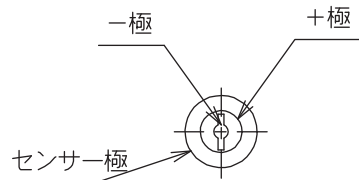
DCプラグ結線図
